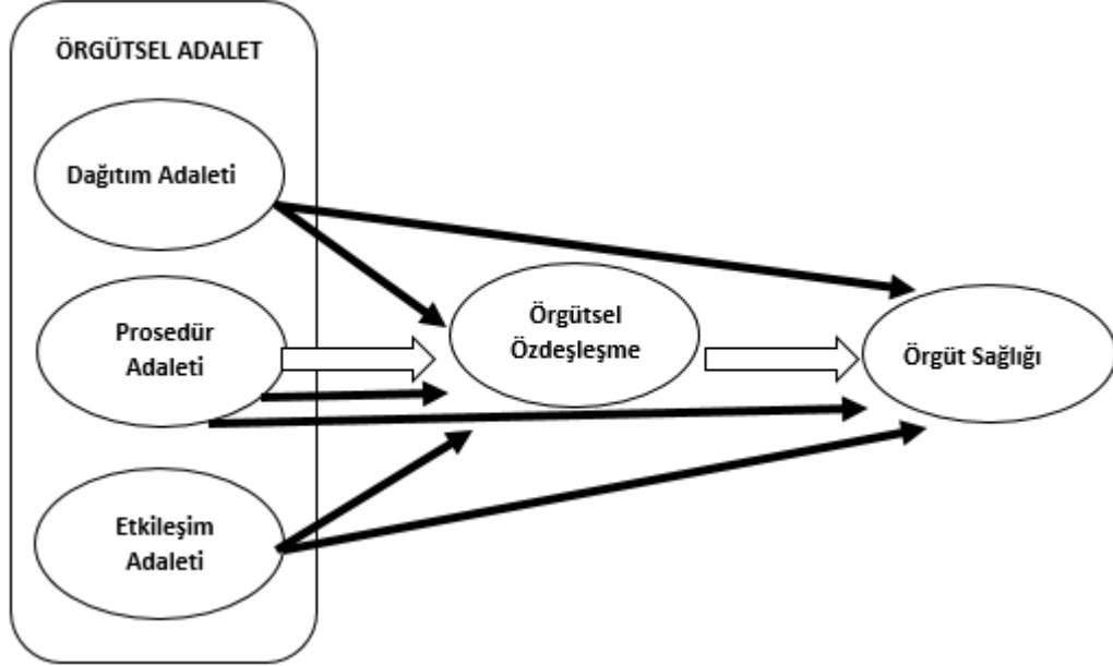
Şekil 4.2. Araştırma Modeli
